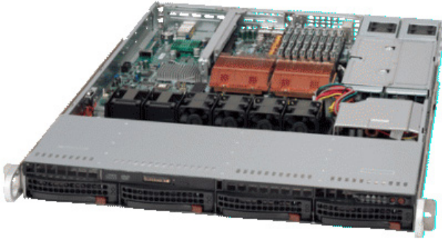
SuperMicro 6016T상세사양
